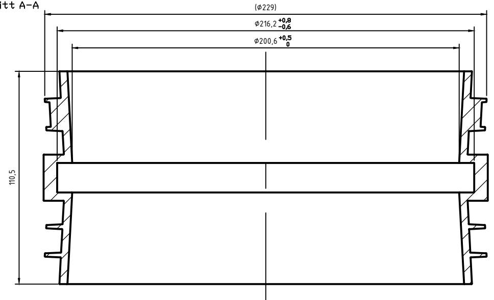
Schnitt A-A
