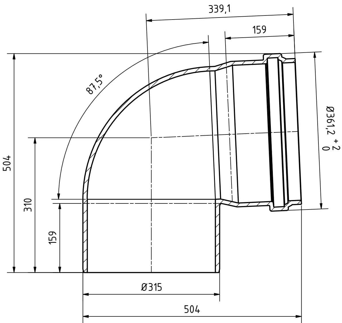
A-A ( 1 : 5 )
