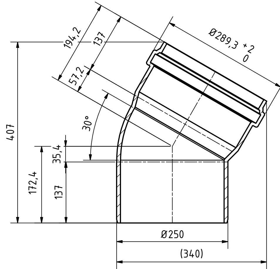
A-A ( 1 : 5 )
