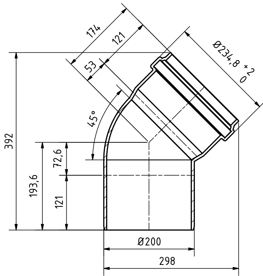
A-A ( 1 : 5 )
