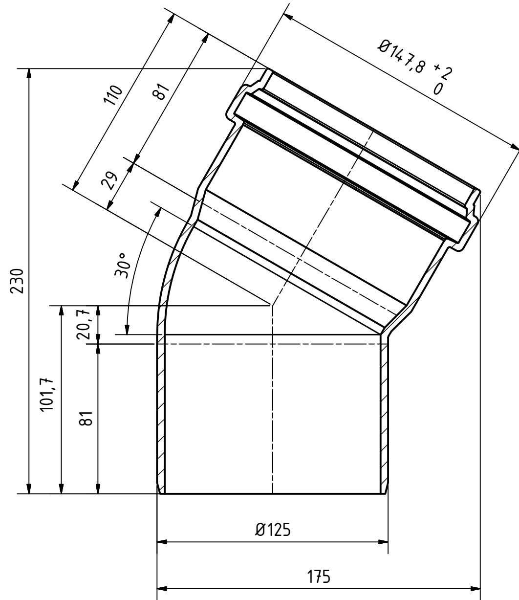
A-A ( 1 : 2 )
