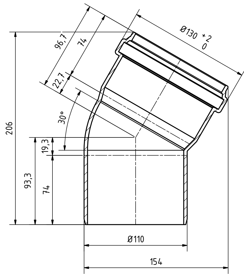
A-A ( 1 : 2 )
