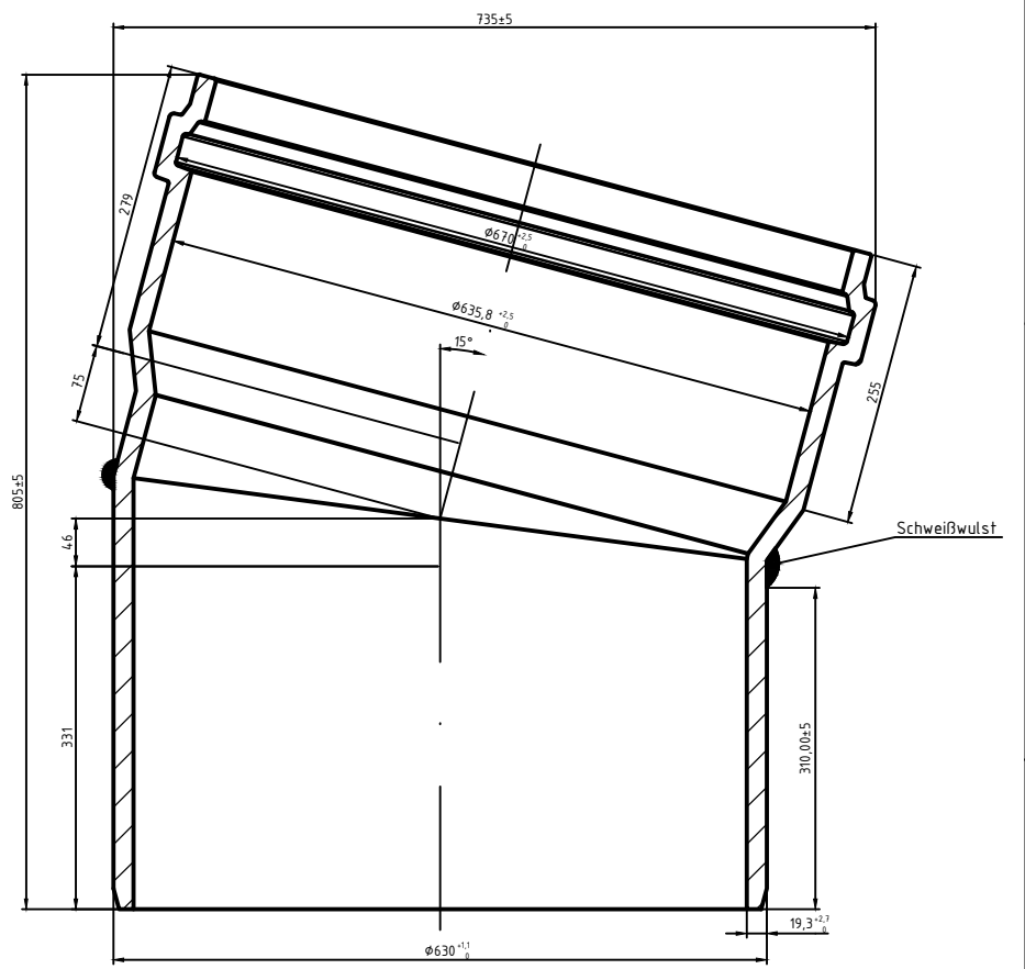
Schnitt A-A
