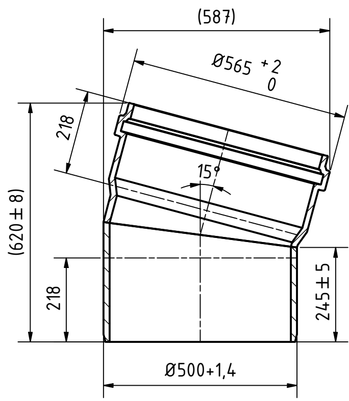
A-A ( 1 : 10 )
