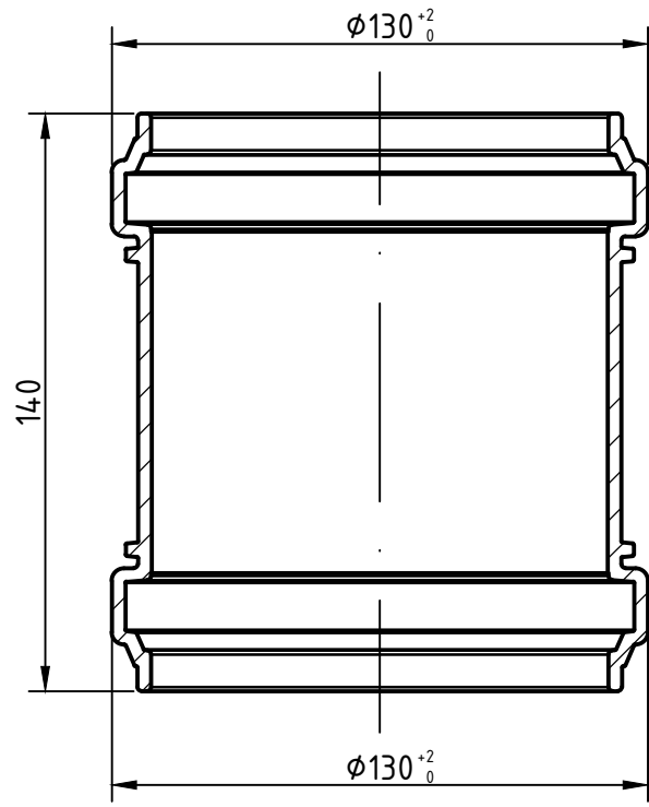
Schnitt A-A
