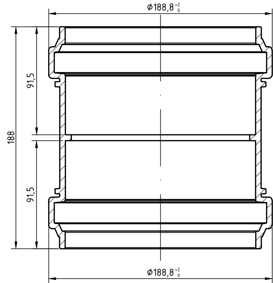
Schnitt A-A
