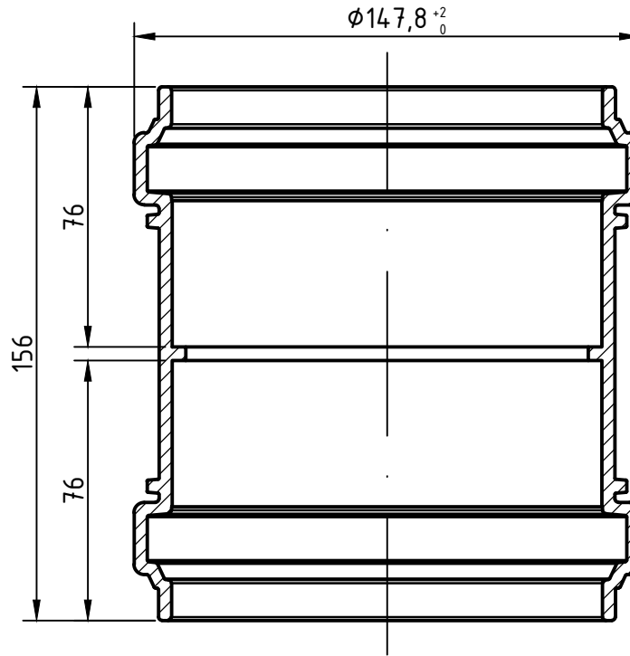
Schnitt A-A
