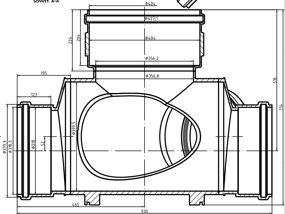
Schnitt A-A
