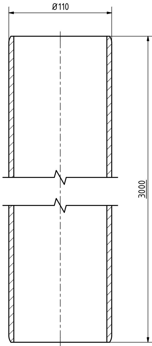
A-A ( 1 : 2 )
