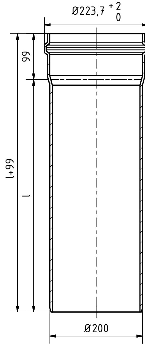
A-A ( 1 : 5 )
