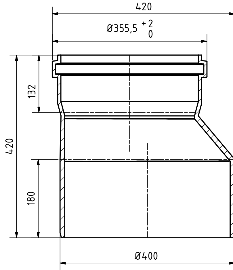
A-A ( 1 : 5 )
