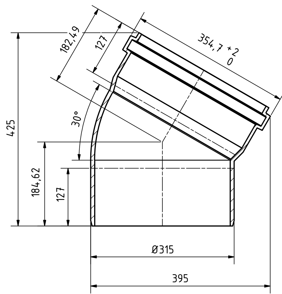
A-A ( 1 : 5 )
