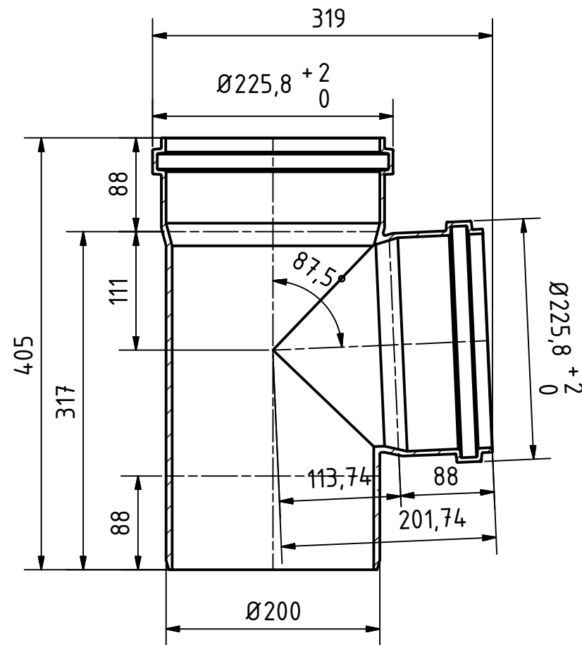
A-A ( 1 : 5 )
