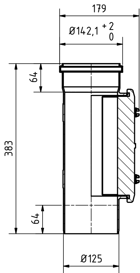
A-A ( 1 : 5 )
