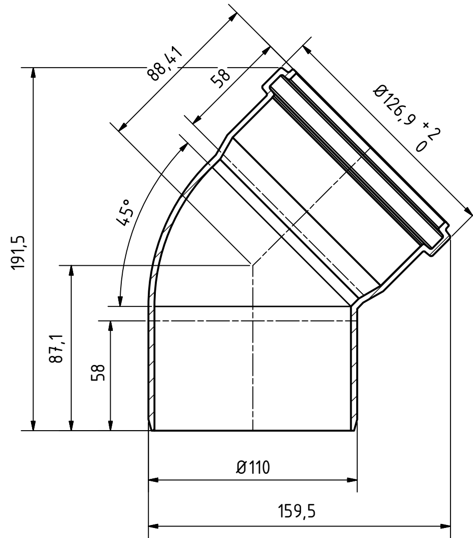
A-A ( 1 : 2 )
