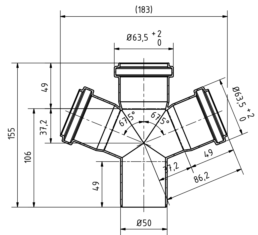
A-A ( 1 : 2 )
